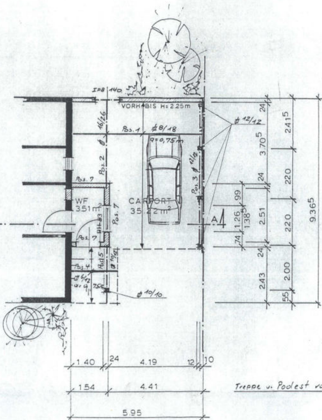
GRUNDRISS
