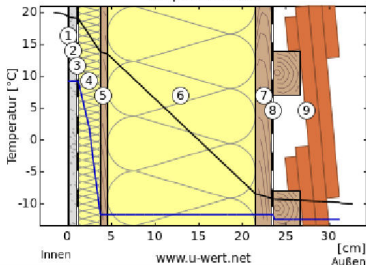
Temperaturverlauf
